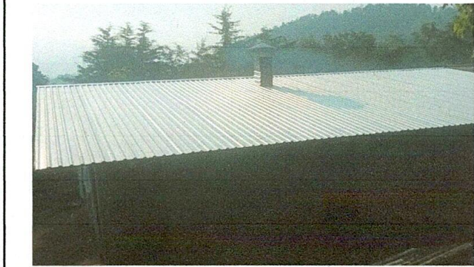
Foto 1: SUTITUCIÓN DE LÁMINAS POR LÁMINAS TROQUELADAS DE CALIBRE 26 , CAPOTES Y TORTILLOS
