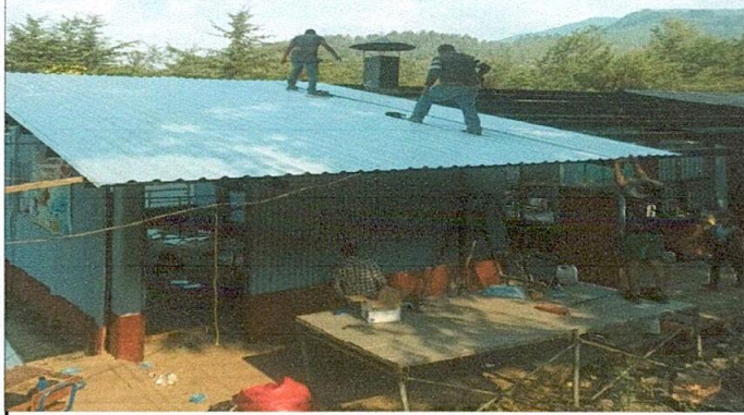
Foto1: SUSTITUCIÓN DE LÁMINAS POR LÁMINAS TROQUELADAS CALIBRE 26, CAPOTES Y TORTILLOS
