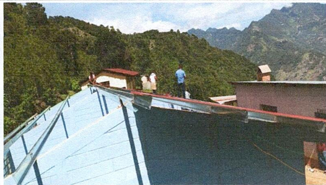
Foto 3: Colocación de costaneras (estructura de soporte)
