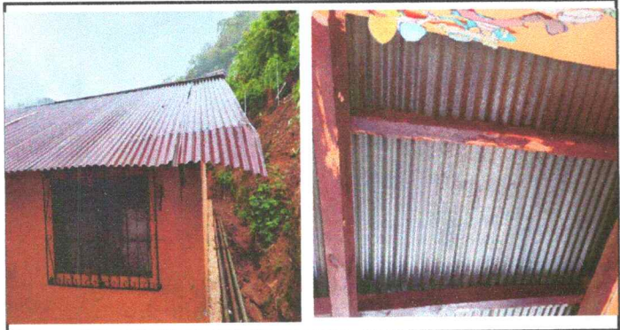
Foto1: Cubierta de lámina y estructura de techo
