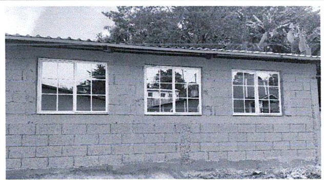
Foto 4: sustitución de ventanas de madera por metal
