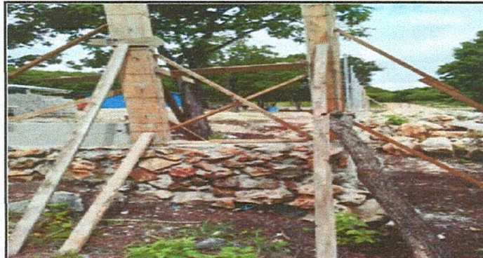
Foto 3: fundición de las columnas o parales donde se colocara la puerta
