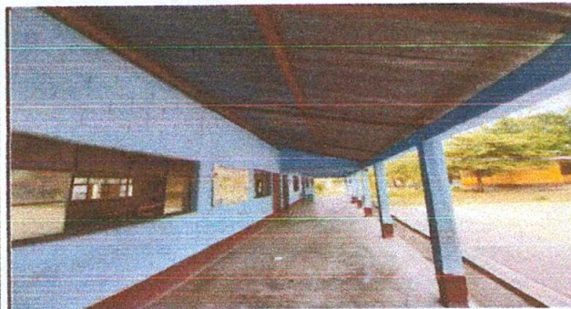
FOTO 5: se pintarán muros interiores y exteriores. Además, sobre la viga principal que está sobre los pilares, se subirá con block una altura aproximada de 60 centímetros por todo el largo del edificio
