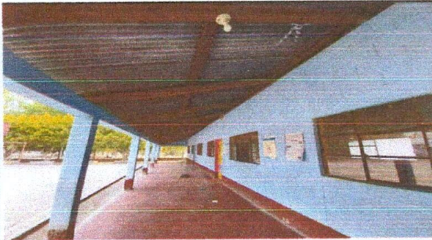
FOTO 3: se sustituirá estructura de madera por metal en 3 aulas. Se ocupará tubo cuadrado de 4 x 4" y tubo rectangular de 3 x 2"
