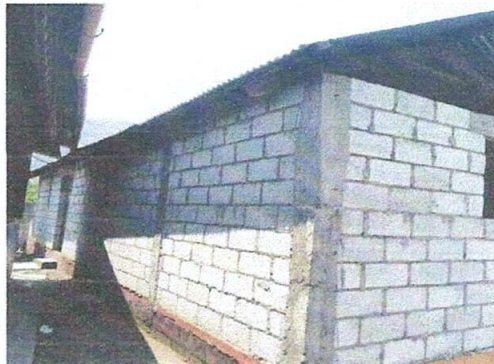
foto 2: Cambio de techo
