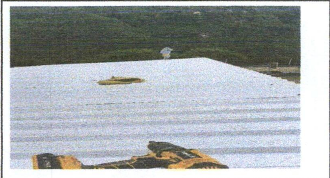
Foto 2: láminas en malas condiciones
