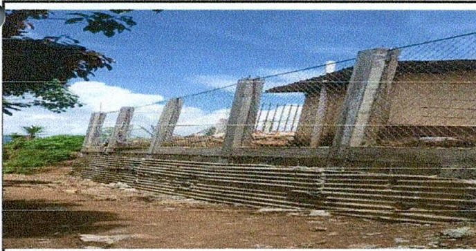
Foto 5. Reparación de muro de concreto finalizado.
