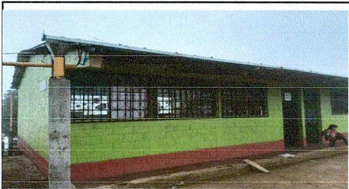
Foto 3. Canaletas instaladas con sus respectivas bajadas de agua con tubos plásticos y pilares de concreto.
