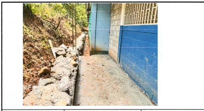
FOTO 5: CONTINUACIÓN DE MURO DE CONTENCIÓN
