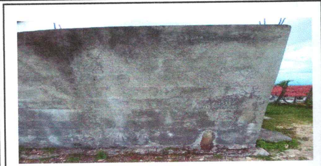
Foto 1: Cisterna de concreto en mal detereorada por completo
