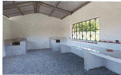
Foto 6: Estufas rurales instaladas y terminadas
