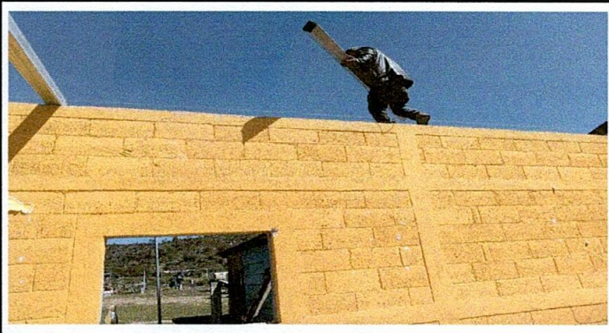
SUSTITUCION DE ESTRUCTURA DE SOPORTE DE TECHO DE MADERA POR METAL
