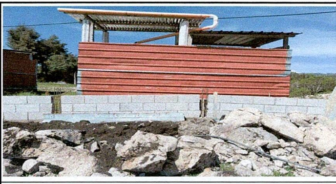
SUSTITUCION DE MURO DE PIEDRA POR MURO DE BLOK, TUBO Y MAYA
