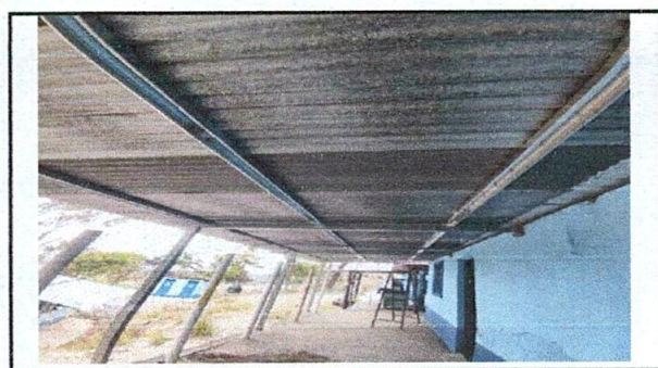
Foto 4: Estructura techo
