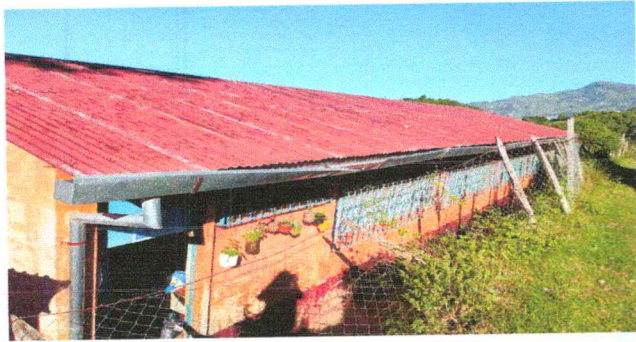
Foto 1: sustitucion de lamina, por lamina troquelada aluzinc calibre 26 y capote
