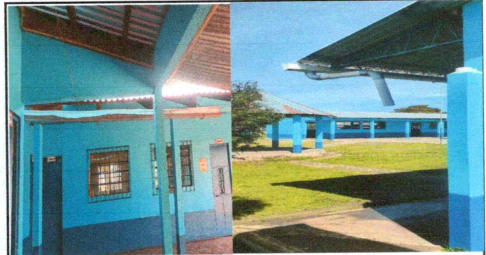
FOTO 8: Sustitución de bajada de agua pluvial de metal por tubo pvc de3*
