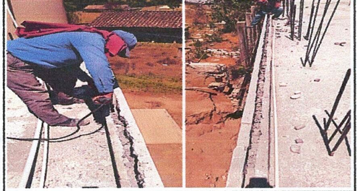
Foto 2: Reparación y mantenimiento de cisternas / depósitos de agua
