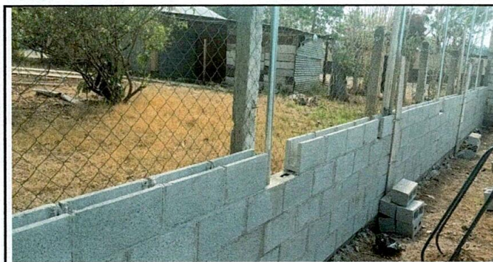
Foto 5: colocación de muro perimetral de block con tubo hg y malla galvanizada, soleras intermedias y columnas.
