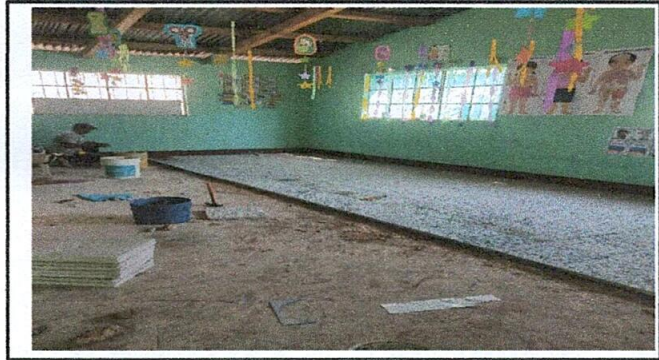
COLOCACIÓN DE PISO EN EL AULA DE PARVULOS SECCIÓN B
