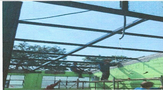
Foto1: Sustitución de estructura de madera, por metal en modulo 1 conformado por un aula y la cocina
