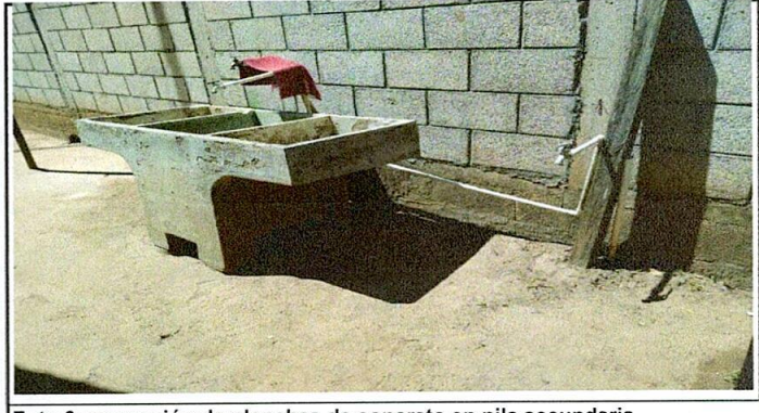
Foto 6: reparación de planchas de concreto en pila secundaria
