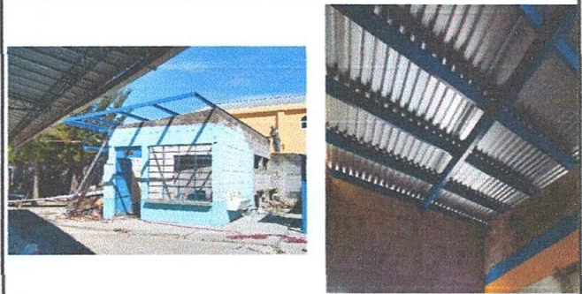
FOTO 2: SUSTITUCIÓN DE LÁMINA Y ESTRUCTURA DE SOPORTE
