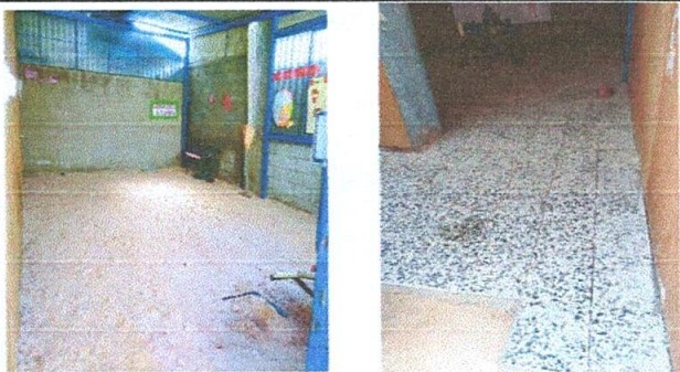
Foto 5: SUSTITUCIÓN DE TORTA DE CONCRETO POR PISO GRANITO
