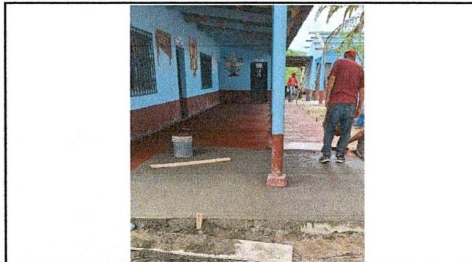
Foto 3 Cambio de tortas de cemento en el corredor
