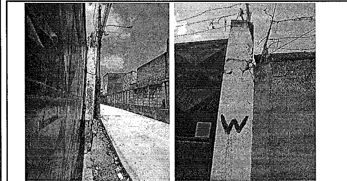
FOTO 3: REPARACION DE COLUMNA, QUE SOPORTA PORTON PRINCIPAL DE 8.50x4.00 MTS.
