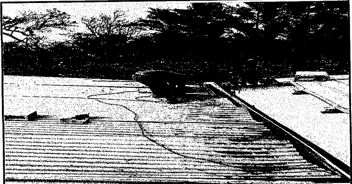
Foto 1: CAMBIO DE LAMINA DAÑADA POR ARENA VOLCANICA ACUMUADA
