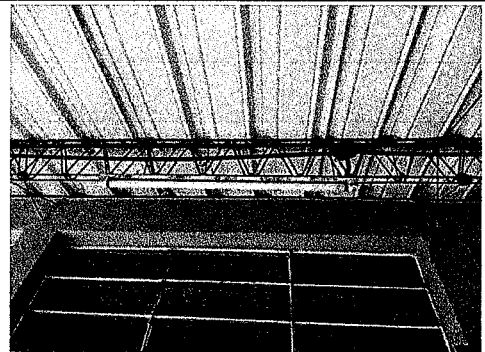
Foto 4: Modulo 17 sustitución de lámparas por lámpara led corredor
