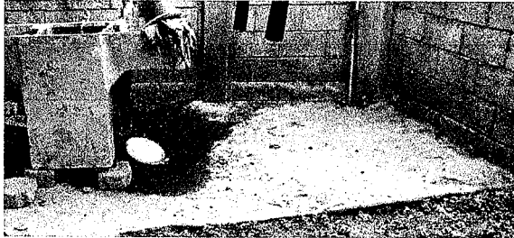
Foto 1: Modulo 16 reparación losa de patio
