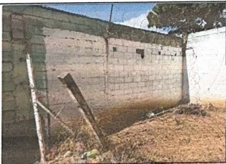
Foto 5: Modulo 1, se observa que necesita repello y cernido
