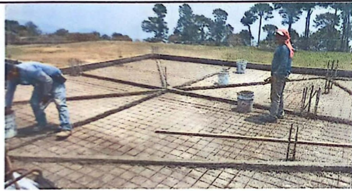
Foto 3: LOSA DAÑADA NO CUENTA CON PAÑUELOS Y CUENTA CON FISURAS, LAS CUALAS OCASIONAN FILTRACIONES DE AGUA, ASI MISMO SE REALIZARAN LOS PAÑUELOS Y SU IMPERMEABILIZACION DE LOSA .
