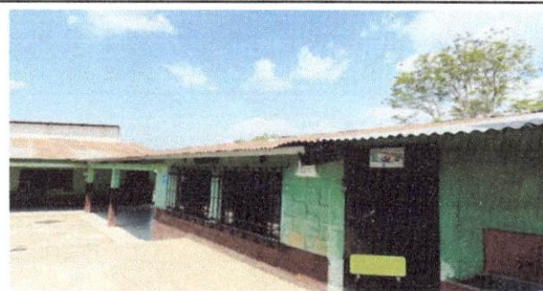
Foto 6: Cambio de estructura de Techo y cubierta de lamina troquelada
