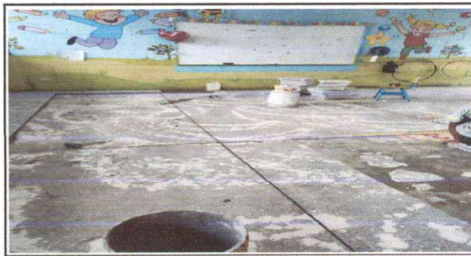
Foto 5: Avance de colocacion de piso
