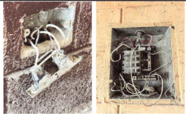
Foto 6: La instalación de tomacorrientes se encuentra en malas condiciones desde el tablero.
