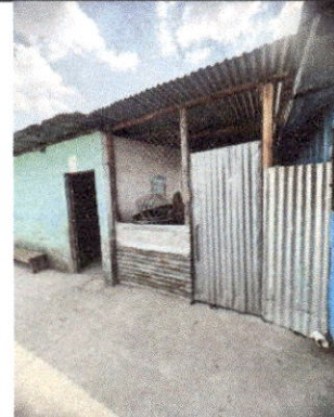
Foto 4: Los muro de cerramiento de la cocina son provisionales por lo que se deberán realizar en block.
