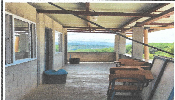
Foto 8: Instalación de Estructura Metálica (segundo nivel)
