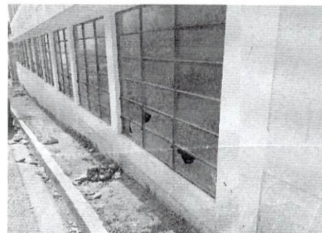
Foto 6: Balcones para ventanas en la parte exterior del establecimiento para seguridad del mobiliario y documentos en aulas
