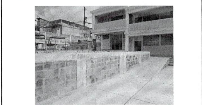
Foto 8: Reparación de muro de contención que representa un peligro para los alumnos del nivel preprimaria
