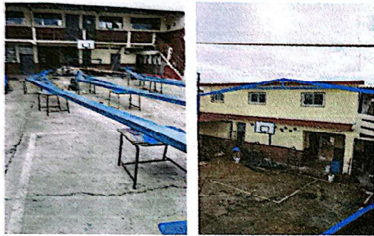
Foto 7: Fabricación de tijeras para techo + instalación de las mismas.
