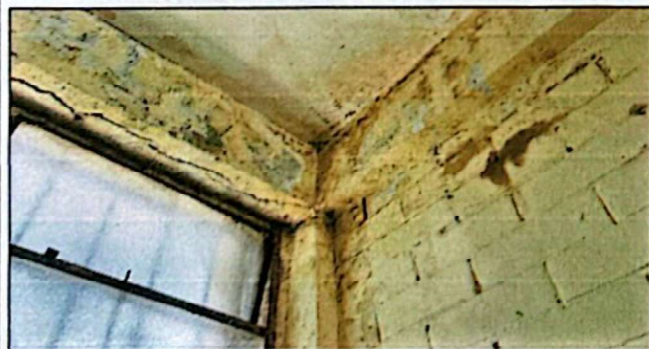
Foto 5: Reparación de 1 Viga en mal estado
