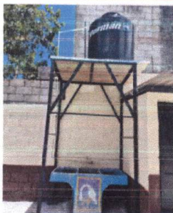
Foto 11: Instalación de tinaco de 1100 litros.
