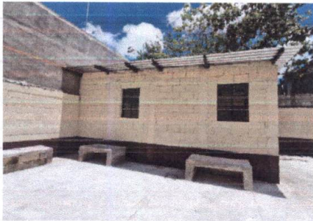
Foto 5: Cambio de techo, mantenimiento de costaneras, colocacion de pisos y ventanas.
