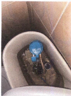
Foto 9: sustitución de accesorios a inodoro
