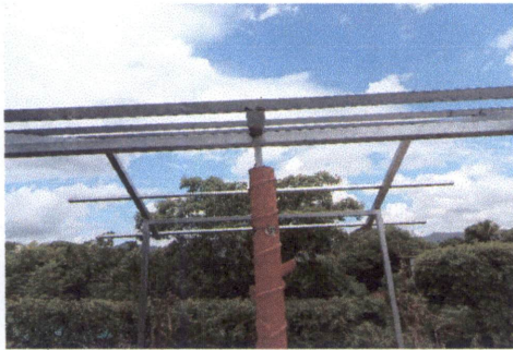
FOTO 1: SUSTITUCIÓN DE ESTRUCTURA DE SOPORTE DE MADERA POR METAL, FALTA INSTALACIÓN DE LÁMINA TROQUELADA CALIBRE 26
