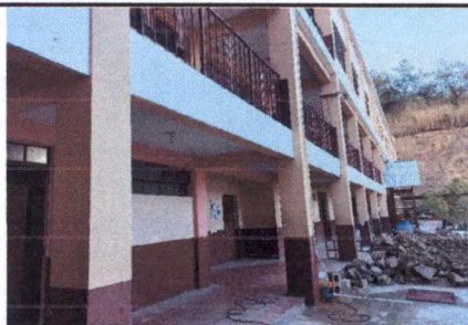
FOTO 6: INSTALACIÓN DE TUBERÍA DE AGUA DESDE CISTERNA HACIA DEPÓSITOS DE AGUA EN TERCER NIVEL
