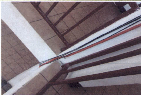
FOTO 5: SUSTITUCIÓN DE DUCTO Y CABLEADO ELÉCTRICO
