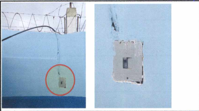
Foto 8: Sustitución de acometida eléctrica, cambio de bases en caja socket, tablero rh, flipon principal de 2*40amp, cable no. 6, tablero de 8 circuitos y 6 flipones.
