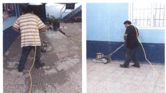
Foto 4: 6 PISO Mantenimiento de piso de granito (pulido y lustrado)
