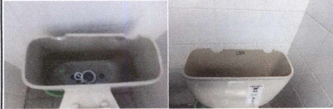
Foto7: 10 SERVICIOS SANITARIOS Y SUS ACCESORIOS Sustitución de accesorios inodoro (contra llave, tubo de abasto y tanque).
