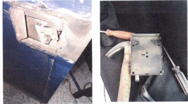
Foto 2: 4. PUERTA DE METAL Sustitución de Chapa
