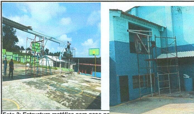
Foto 2: Estructura metálica para paso peatonal.
