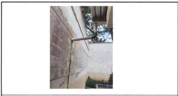
Foto 17: Reparación de bajada de agua en área de patio, se colocará directa hacia el patio.
