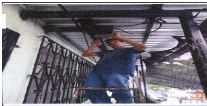
Foto 5: Instalación de tablero de cuatro polos, cableado y empalmado.
