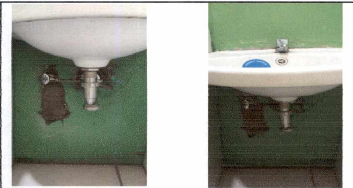
Foto 9: Reparación de fuga en lavamanos
