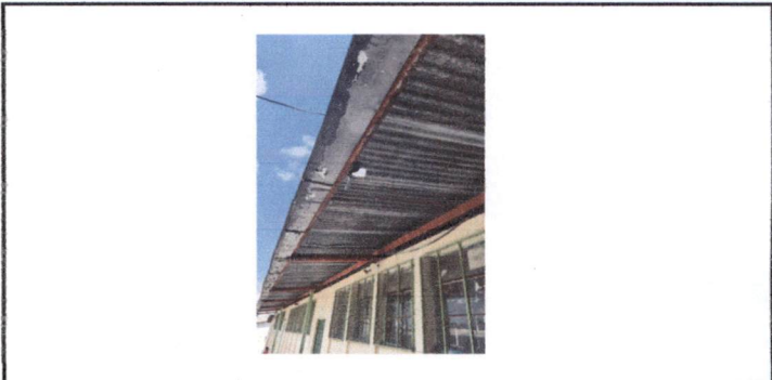
Foto 2: Módulo 1 de aulas. Lámina de pasillo con agujeros, deteriorada y en mal estado, presenta filtraciones
