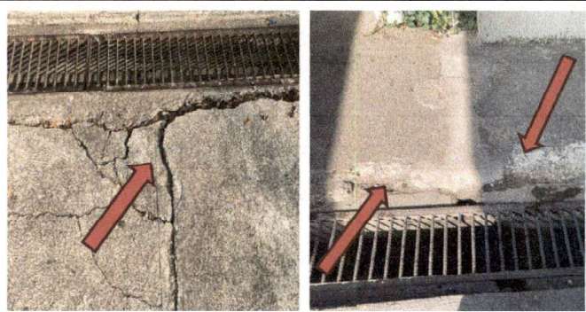
Foto 7 y 8: 8. CUNETA DE CONCRETO 8.1 Reparación de cuneta de concreto
