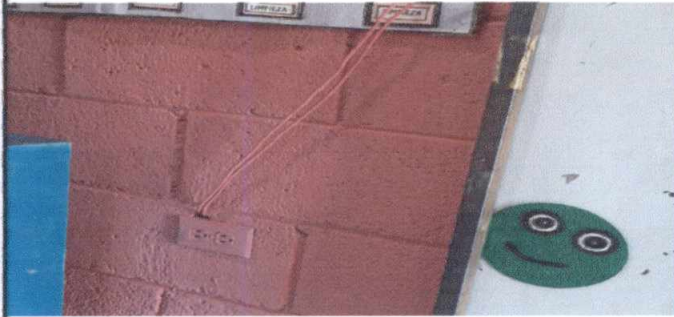
Foto: 13 sustitución de tomacorrientes dobles
